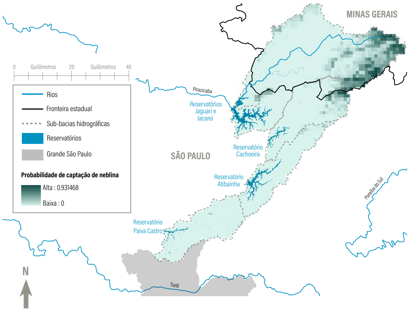
Figura 7 | Probabilidade de ocorrência de floresta nublada no Cantareira (representa a captação de neblina)
