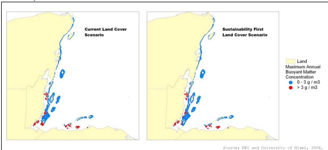
Figura 13. Mapa de la Concentración de Materia Suspendeda en el Arrecife Mesoamericano (Escenarios de Cobertura Terrestre Actual y Sustentabilidad Primero)
